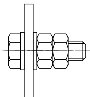
A-A (1:1)
